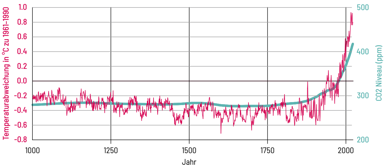
Grafik 13: Gleichzeitiger Anstieg der weltweiten CO 2 -Emissionen (ppm) und der Mediantemperatur (in °C im Vergleich zu 1961–1990) (Quelle: Meinshausen et al. 2017 ; Neukom et al. 2019 ; Climatic Research Unit (University of East Anglia) and Met Office 2023 ).
