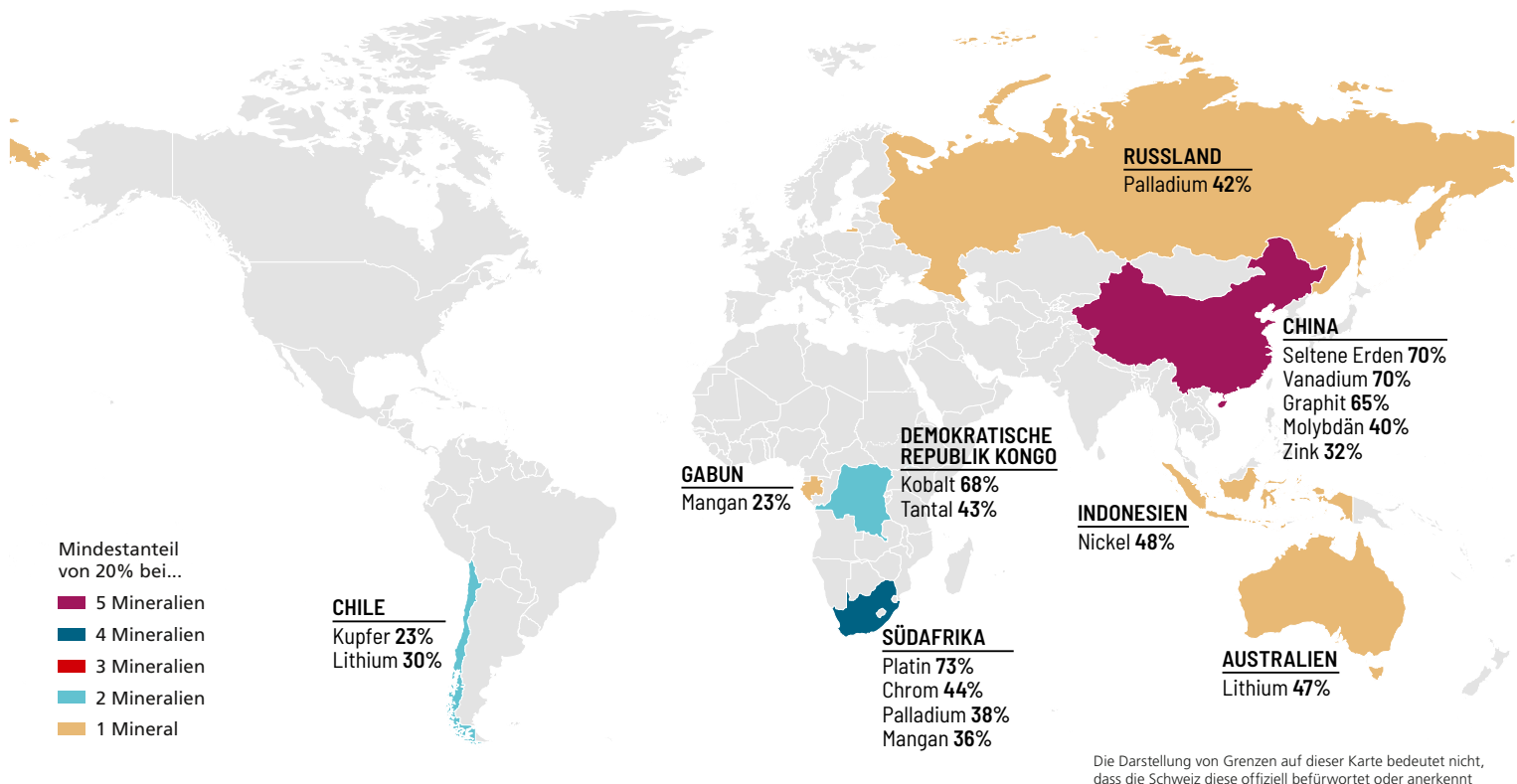
Grafik 4: Geografische Konzentration des globalen Abbaus von Mineralien, die für die Energiewende wichtig sind (Quelle: U.S. Geological Survey ).
