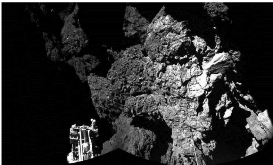
© ESA/Rosetta/Navcam
